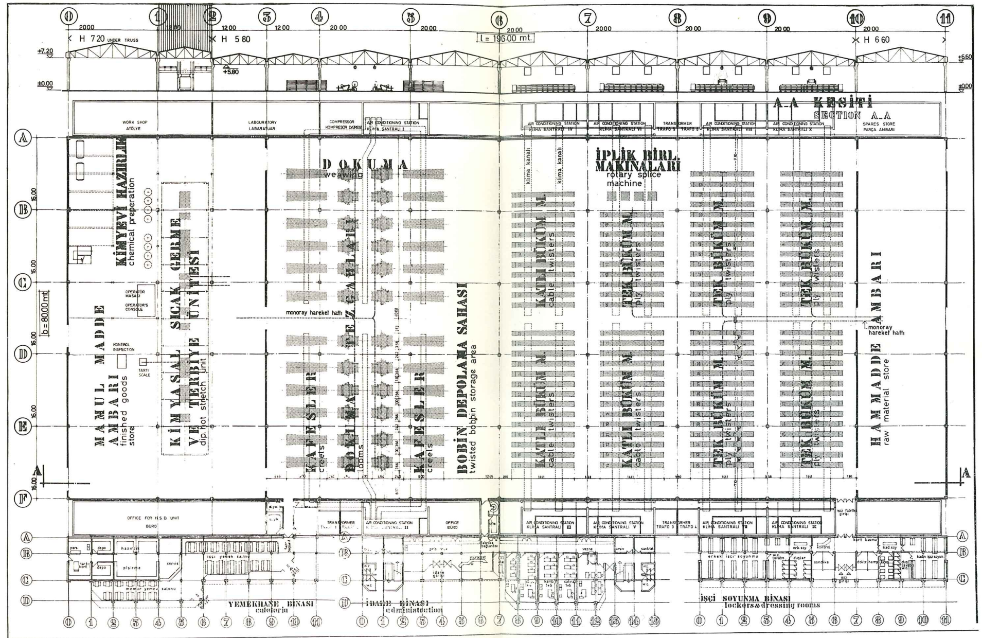
KORDSA KORD BEZİ TESİSLERİ GENEL DİZPOZİSYON PLANI
